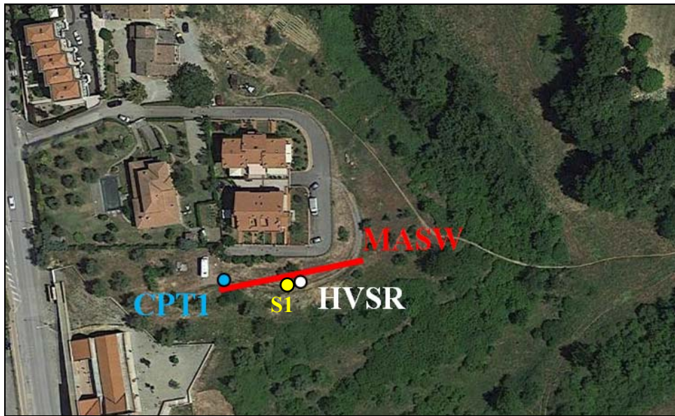
Fig. 4 - profilo indagato tramite prova sismica (scala indicativa)
